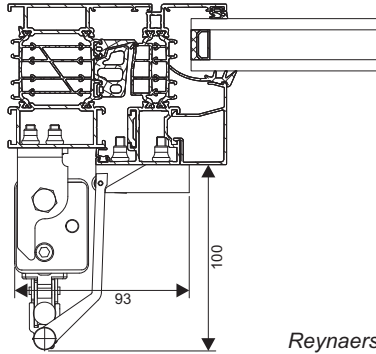
Reynaers® CS86HI
